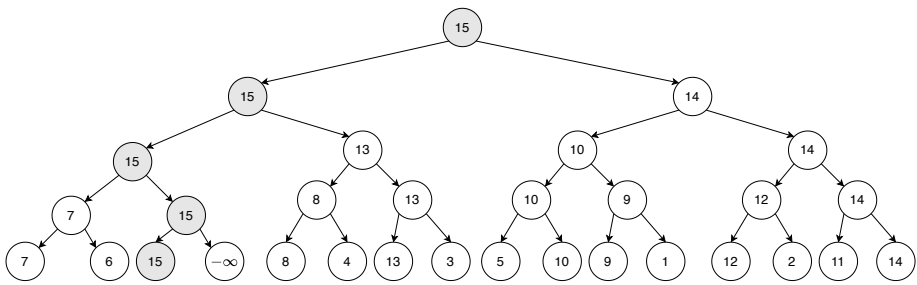
取出 16, 将其替换为 -\infty , 15 上升为新的根
