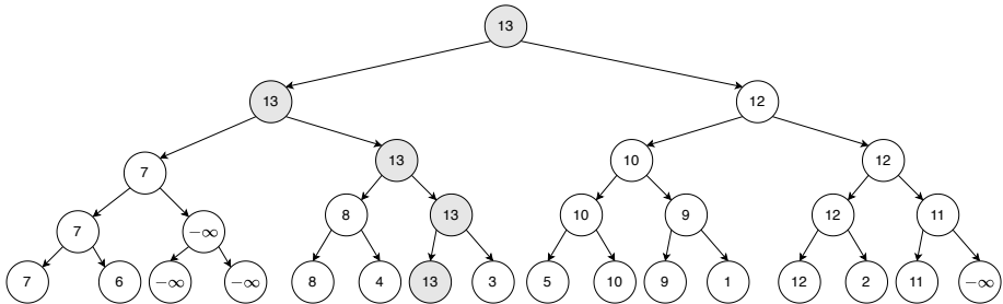
取出 14, 将其替换为 -\infty , 13 上升为新的根
