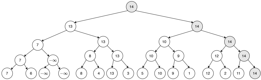
取出 15, 将其替换为 -\infty , 14 上升为新的根
