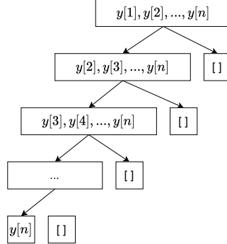
(b) [y_1 > y_2 > \dots > y_n] 的划分树, ≥ p 的部分总为空。
