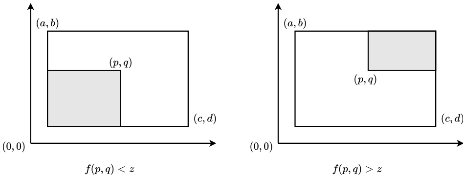
(a) 如果 f(p, q) \neq z , 只能丢弃左下或右上的灰色区域, 剩余区域变成了 L 形。
