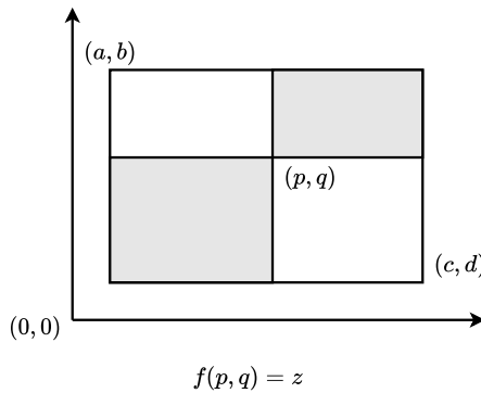
(b) 如果 f(p, q) = z , 可同时丢弃两个灰色部分, 搜索区域减半。
