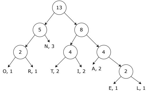
图 15.20: 哈夫曼树
