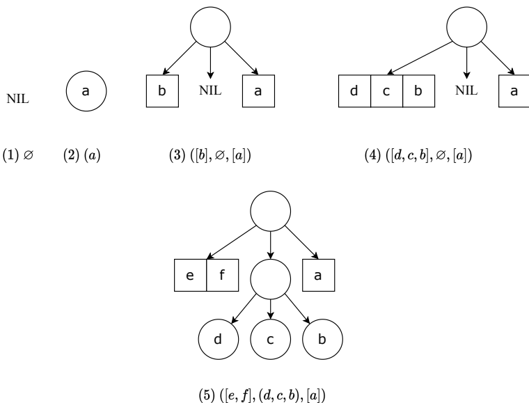
图 12.7: 手指树
