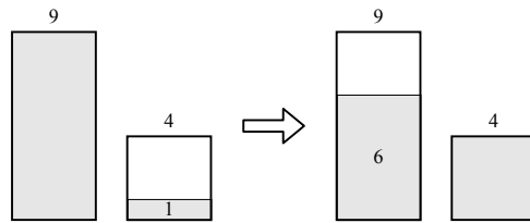
图 15.11: 最后两步
