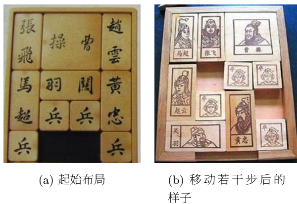
图 15.14: 华容道游戏
