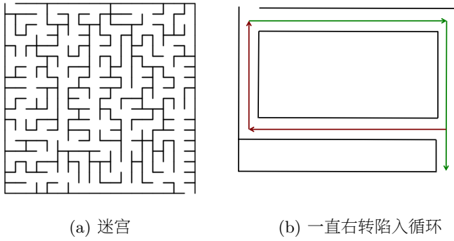
图 15.1: 迷宫
