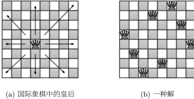
图 15.3: 八皇后问题
