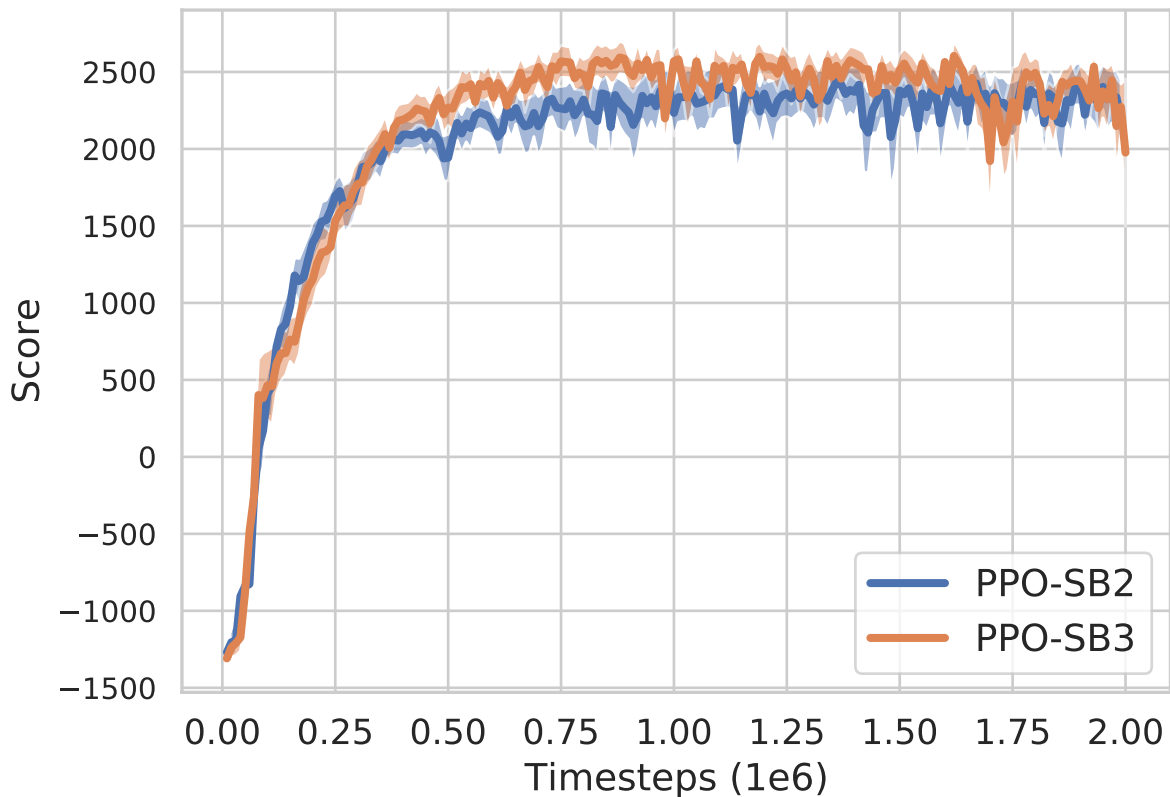
HalfCheetahBulletEnv-v0
